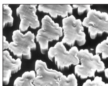
Querschnitt einer „No Name“ Viskose aus Asien
