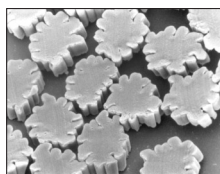
Querschnitt von SULKY aus 100% ENKA Viskose
