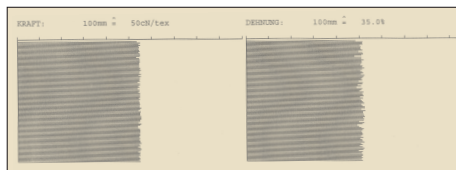
SULKY Viskose im Kraft- und Dehnungstest: hohe Gesamt Reißkraft
